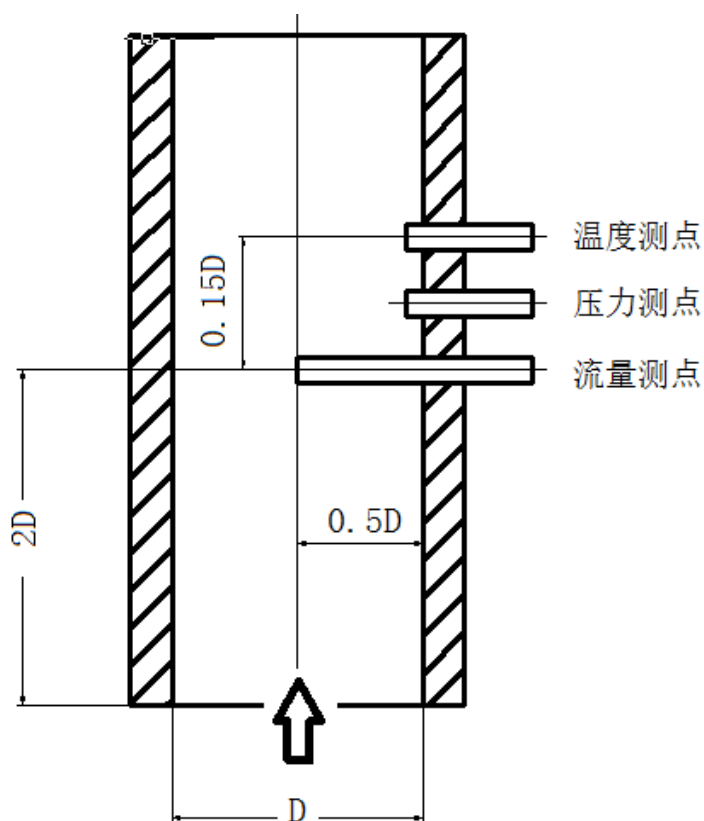
图1 燃料管道测点布置
