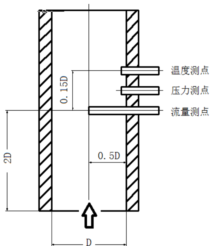
图2 空气管道测点布置
