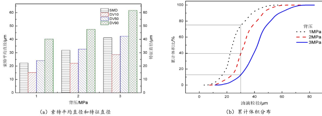
图5 不同喷口直径条件下喷雾雾化特性
