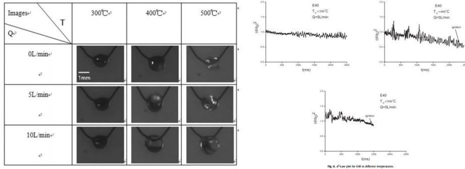
图4.不同温度及气体流量条件下生物柴油和乙醇燃料的着火和微爆特性
