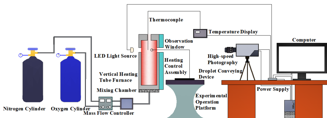
图3基于运动图像跟踪技术的液体混合燃料微爆特性测试方法原理
