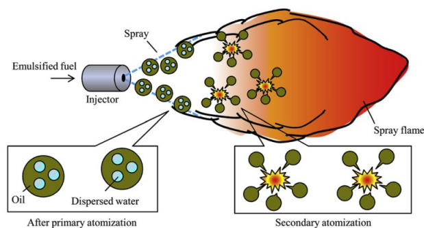
图2. 混合燃料液滴的微爆和二次雾化原理
